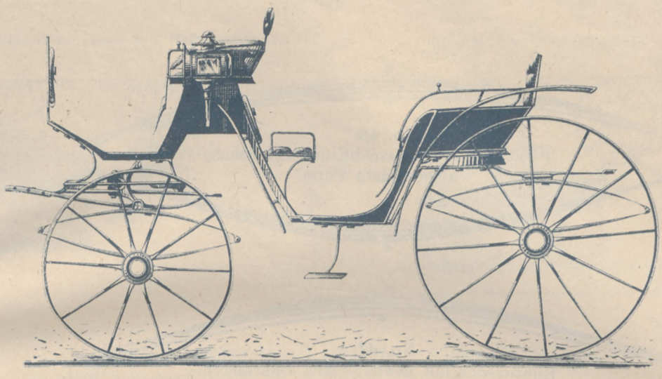
Familien-Phaëton (Tafelwagen.) No. 12.
