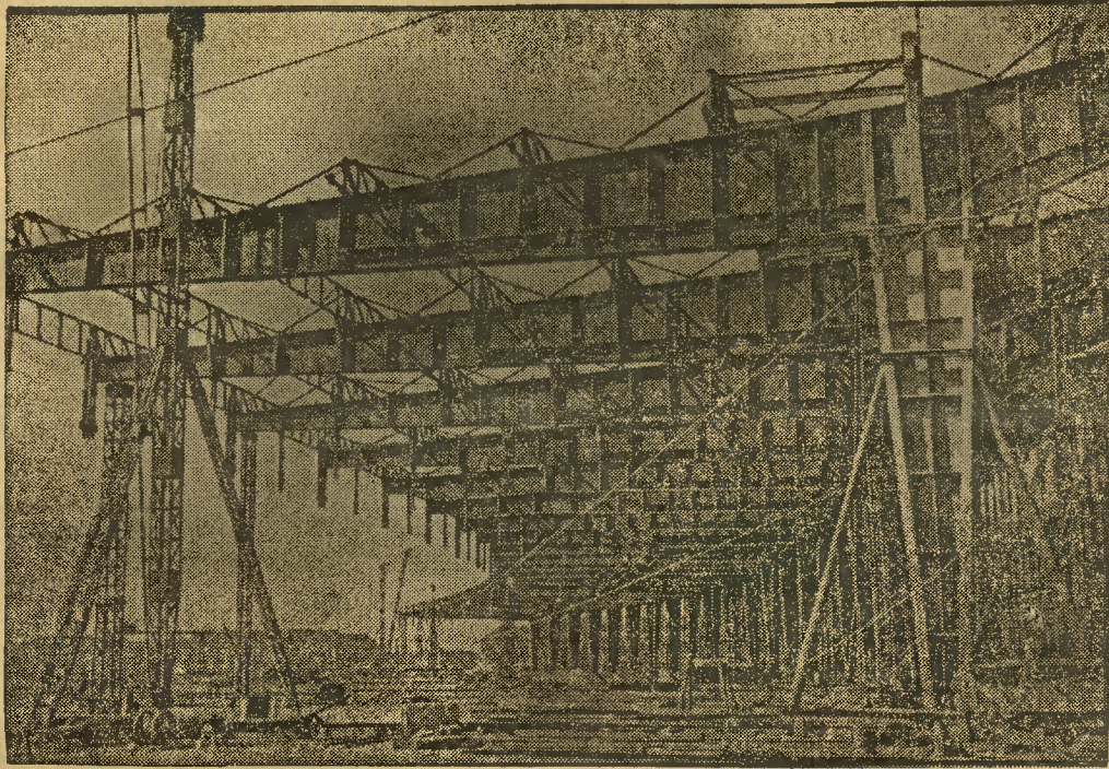
Na berlińskim Tempelhofie buduje się największe lotnisko na świecie. Na zdjęciu: konstrukcja stalowa nowego olbrzymiego hangaru.
