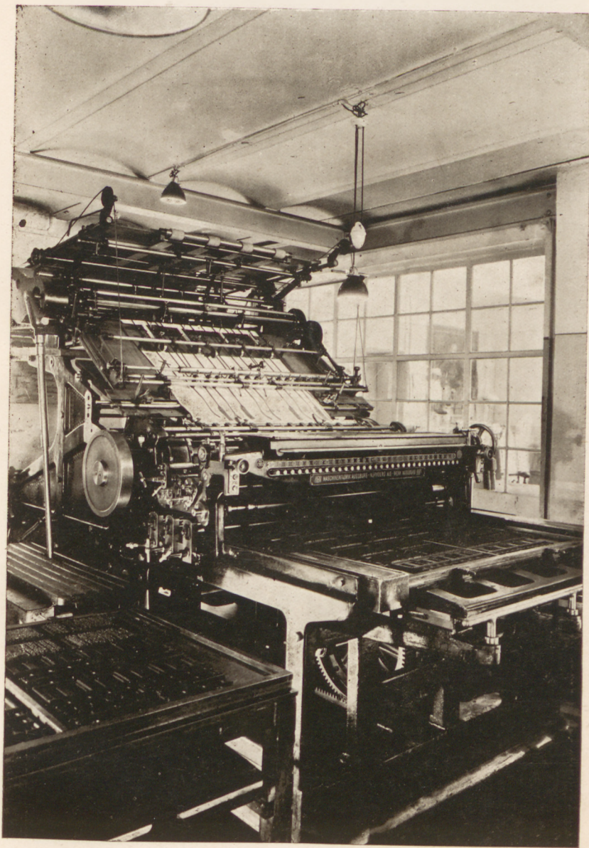
Nowoczesna maszyna pospieszna do druku z samonakładaczem »Rotary«
