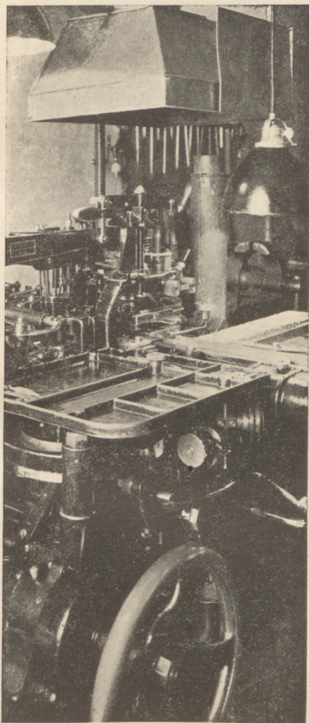
Angielska maszyna odlewnicza »Monotype«
