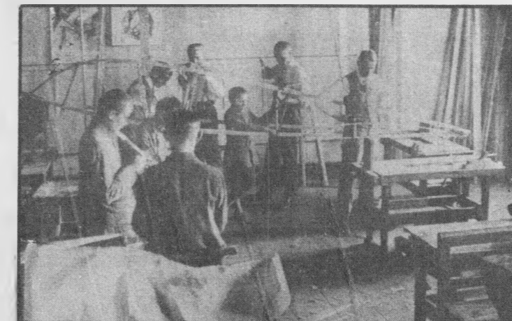
Szkoła modelarska przy Gimnazjum im. Staszica w Lublinie: 1) Kurs modelarski klas młodszych. 2) Szkielet przyszytych szybowców. 3) Uczniowie przy budowie skrzydła szybowca.
