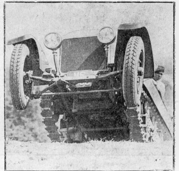
Nowy typ czołgu bojowego, posiadany przez Armię Angielską.
