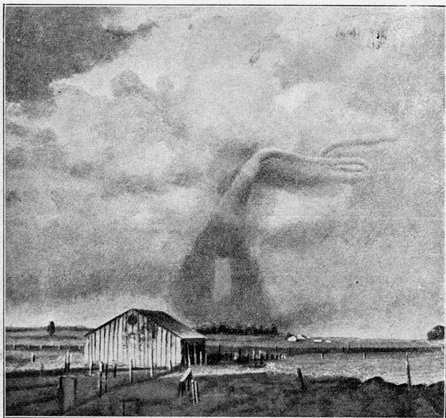
Niezwykle interesującą fotografję cyklonicznej trąby powietrznej udało się uchwycić w Minnesota w Stanach Zjednoczonych.
