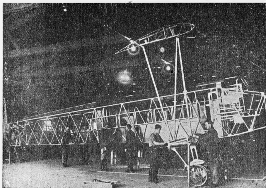
Budowa aeroplanu.
