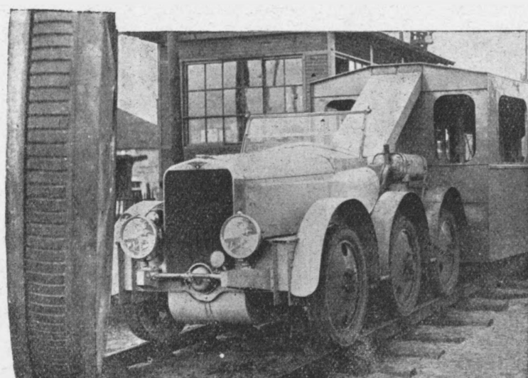
Dokonano we Francji ciekawej próby — zastosowania opon gumowych do sprzętu kolejowego o napędzie benzynowym. Próby dały znakomity wynik, przy czym stwierdzono, że 300-konny silnik daje możliwość rozwinięcia szybkości 140 km. na godzinę.
