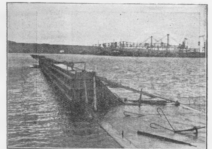
Tama w Gdyni
