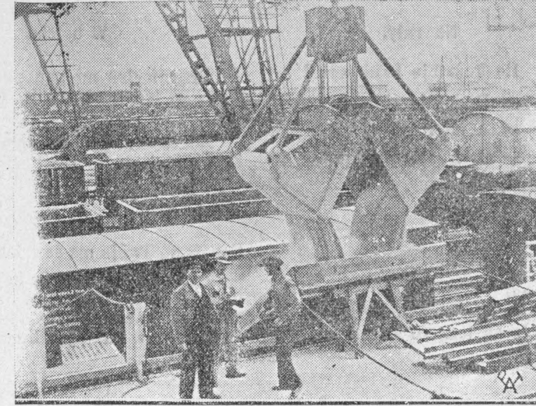
Do portu w Gdyni przybył 1 b. m. na st.tku szwedzkim „S. S. Trolleholm” większy ładunek fosforytu, który w przeciągu kilkunastu godzin — dzięki pomocy potężnego „chwytacza” przeładowany został z okrętu wprost do wagonów, postawionych pod okręt pociągu.
