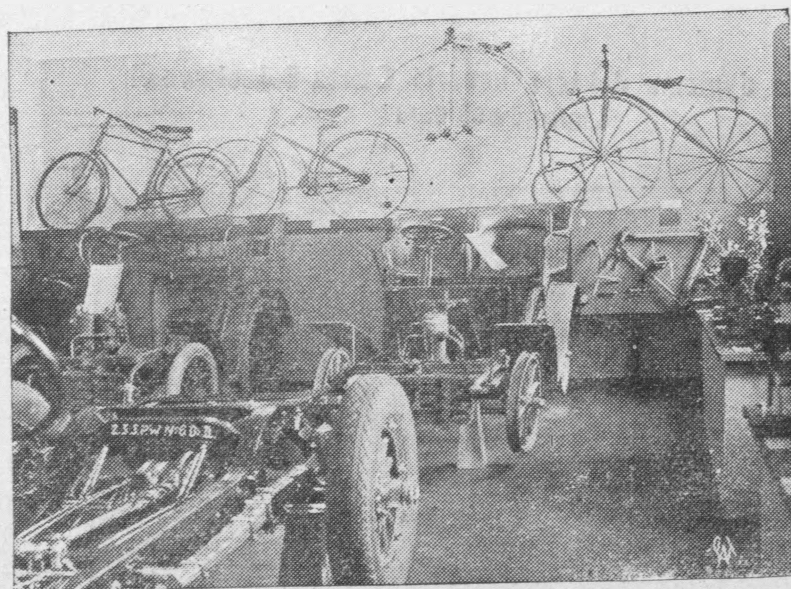
W sobotę odbyło się w Muzeum Przemysłu i Techniki otwarcie dwóch nowych działów, a mianowicie działu Higieny i Bezpieczeństwa Pracy, oraz Historii samochodu. Na zdjęciu — jedna z nowotworzonych sal Muzeum, zawierająca eksponaty przedstawiające rozwój samochodu, poczynając od rowerów, a kończąc na najmniejszych Buickach, Fiatach itp.
