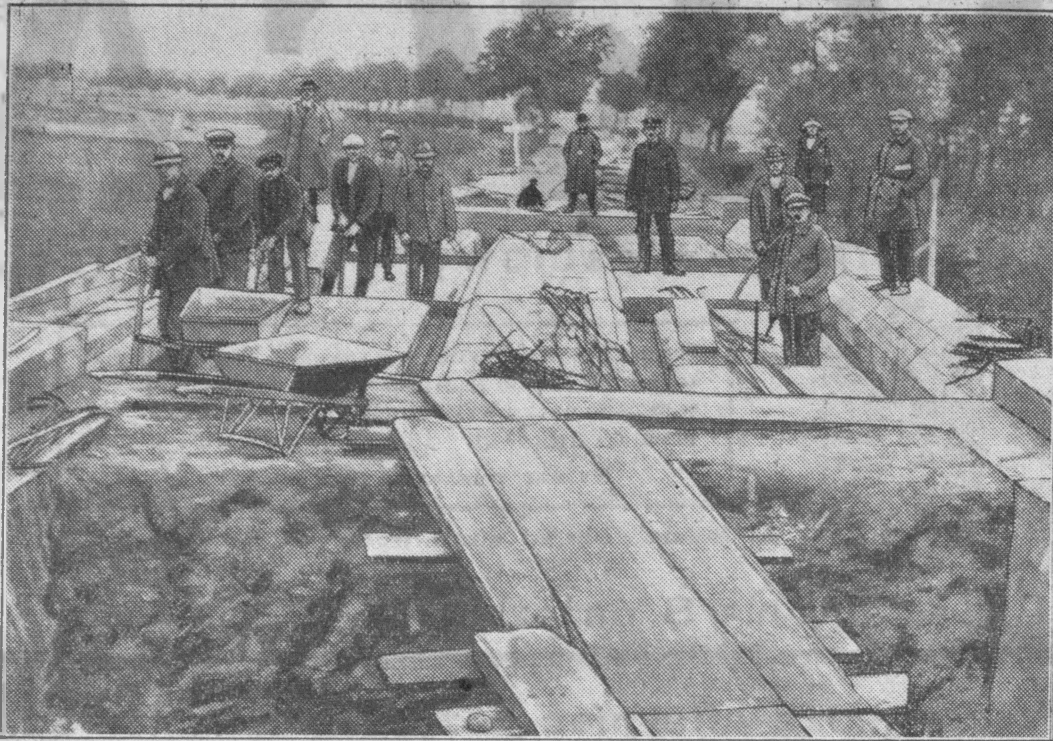
Zaszalowanie do belek, płyty i chodnika.
