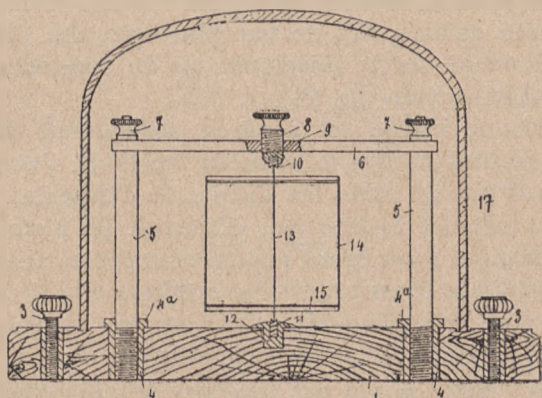
Fig. 20. — Coupe de l'appareil Fayol.
