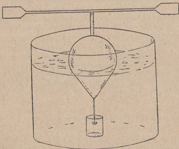
Fig. 22. — Appareil à flotteur.
