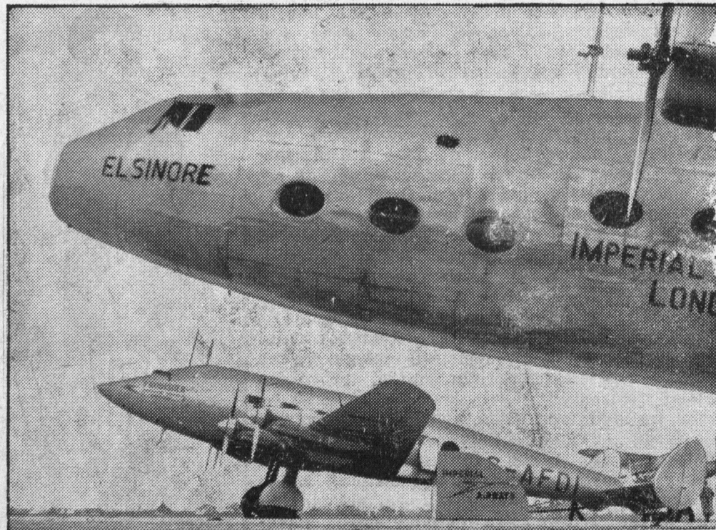
Olbrymi samolot, widoczny na zdjęciu, przebywa trasę Londyn—Paryż w ciągu 64 minut. Samolot ten ma 4 silniki, waży 15 ton i przewozi 22 pasażerów.
