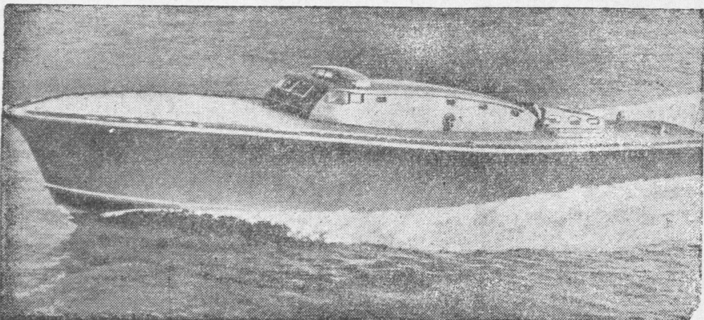
Na wodach wyspy Wight odbyły się próbne jazdy angielskiego torpedowca najnowszej konstrukcji. Torpedowiec długości 25 m, o sile 3 motorów 1000 KM, rozwija szybkość 50 mil morskich na godzinę. Łódź jest wyposażona w 2 wyrzutnie torpedowe 53 cm albo w 4 wyrzutnie o kal 45,75 cm, w srmatkę i bomby głębinowe oraz w aparat do wytwarzania sztucznej mgły.
