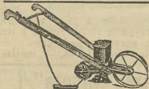
Siewnik L. 3 . Wysiewa kupkowo różne nasiona: grochy, kukurydzę tępiny, bur-ki i inne nasiona. Skrzynka jest pojemności 3 litr. Koło biegowe ma 28 cm. Komplet zł 95,-
