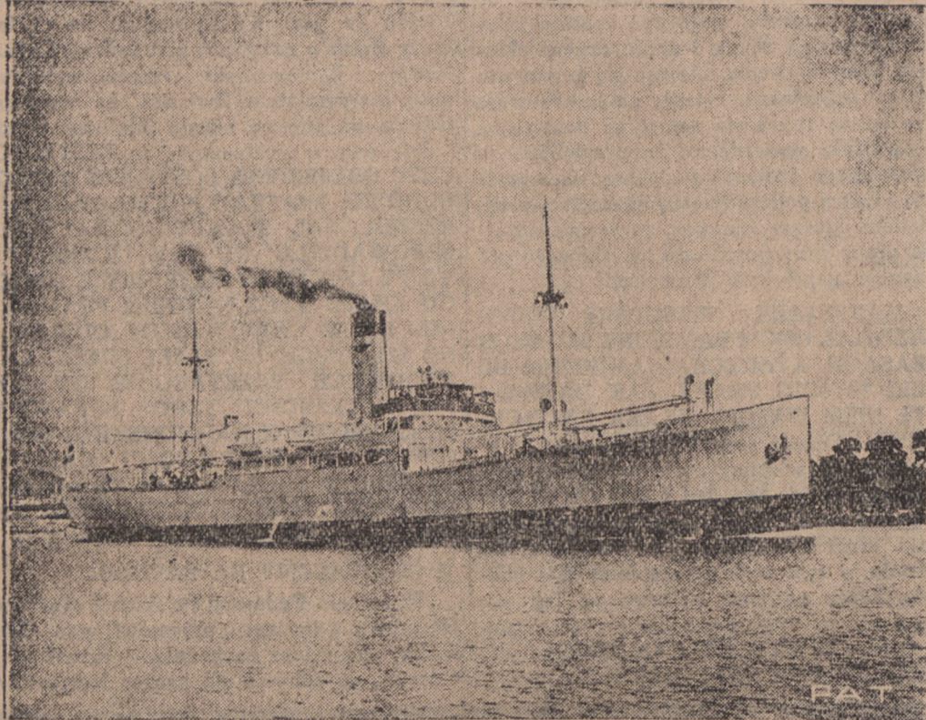
Do portu w Gdyni zawinął najnowszy statek żeglugi polskiej s.s. „Lwów“, wybudowany w stoczni duńskiej w Helsingör, dla polsko-brytyjskiego towarzystwa okrętowego. — „Lwów“ jest bliźniaczym statkiem s.s. „Lublin“, odebranego przez polsko-brytyjskie towarzystwo z tej samej stoczni już przed kilku tygodniami. s.s. „Lwów“ posiada pojemność 1.308 tonn reg. brutto. Jest on wyposażony w nowoczesne chłodnie i przeznaczony do przewozu ładunków produktów spożywczych. Statek ten kursować będzie regularnie raz na tydzień na linii Gdynia — Gdańsk — Hull. Na ilustracji naszej widzimy podobiznę s.s. „Lwowa“.
