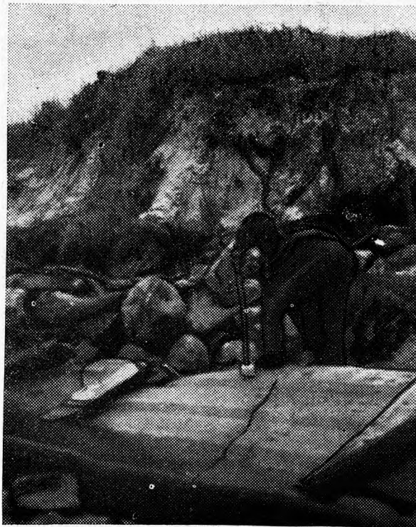
Reprodukujemy olbrzymią wyrwę utworzoną przez burzę na morzu polskim w tamie holenderskiej pod Karwią. Oslona betonowa została rozbita przez szalejący żywioł.
