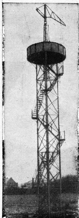
PIERWSZA NA WOŁYNIU WIEŻA SPADOCHRONOWA Na zdjęciu — pierwsza na Wołyniu wieża spadochronowa L. O. P. P., wybudowana w Kowlu, ze składek pracowników kolejowych Dyrekcji Radomskiej P. K. P.
