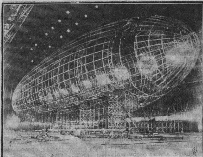
Na zdjęciu naszym widzimy szkielet statku „Akron” w hangarze.
