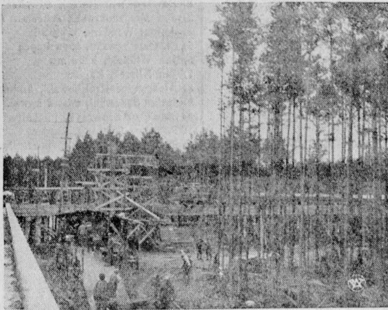
Budowa żelazobetonowa hali fabrycznej w Wysokopiennym lesie sosnowym.
