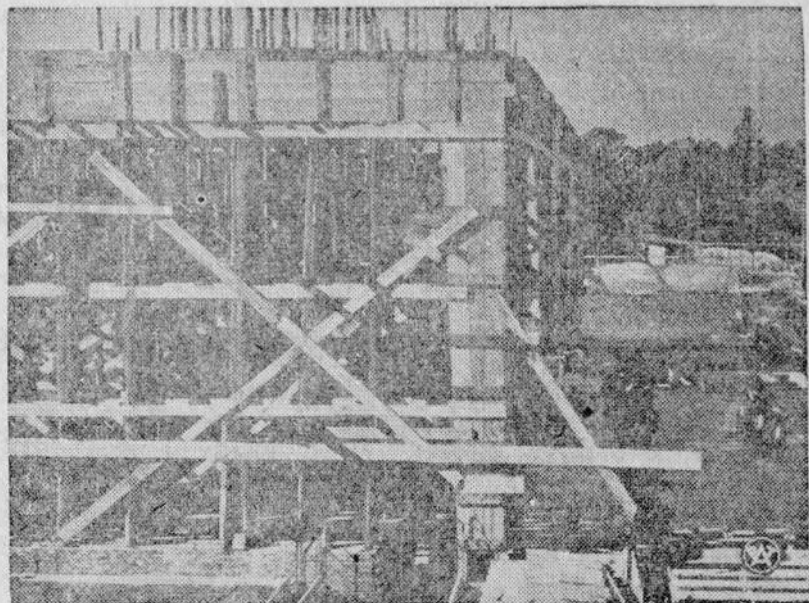
Fragment z budowy: deskowanie stropu hali budynku mechanicznej stacji doświadczalnej we Lwowie.
