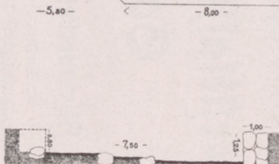
Längsschnitt zur Kapelle.
