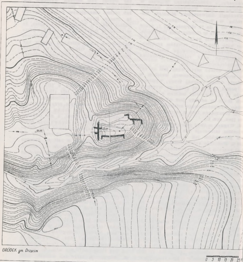
Ryc. 1 — Gródek, gmina Drzycim. Plan warstwicowy z widocznym zarysem bryły zamku
