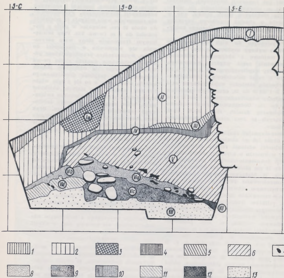
Ryc. 2 — Gródek, gmina Drzycim. Profil północno-wschodni. Legenda: 1 — darń i szary piasek, 2 — jasnobrunatna, silnie spieczona ziemia ze szczątkami organicznymi i węgielkami drzewnymi, 3 — wkop nowożytny, 4 — ciemnożółta, silnie zbita glina z soczewkami rdzawej gliny, 5 — ciemnobrunatna, silnie spieczona ziemia, 6 — ciemnoszara, silnie spieczona ziemia z wtrętami soczewek jasnobrązowej gliny i zaprawy wapiennej, 7 — spalone drewno, 8 — jasnobrązowa, silnie zbita glina, 9 — rumosz spalonej w ogniu gliny i bierwion, 10 — silnie spieczona ziemia zabarwiona spalenizną na kolor ciemnobrązowy, 11 — rdzawy, drobnoziarnisty żwir, 12, 13 — żółty piasek przemieszany z drobnym żwirem
