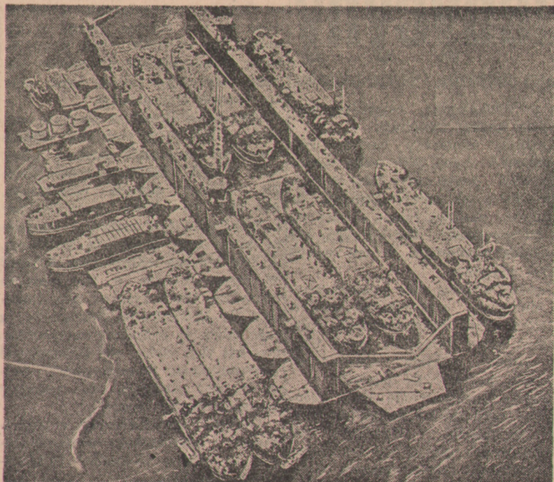
Podczas wojny morskiej na Pacyfiku Amerykanie używali kilku sztucznych portów i piętnastu olbrzymich dźwigów i stocni pływających o ogólnej nośności 1.200.000 ton. Nowoczesne te dzieła techniki wyposażone były we wszelkie urządzenia do naprawy okrętów. Na zdjęciu jeden z takich dźwigów, którego zdolność naprawy okrętów określa się liczbą 100 tys. ton. Dok ten, jak ilustruje to zdjęcie, wyzyskiwany jest i obecnie. W naprawie znajduje się w tej chwili osiem okrętów wojennych i kilka mniejszych jednostek.
