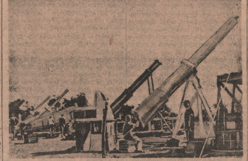
Ostatnie całkowite zaciemnienie słońca najlepiej było widoczne w Brazylii. Tam więc ustawiła swe teleskopy ekipa naukowa ze Stanów Zjednoczonych Ameryki Północnej. Ustawione w szeregu ogromne teleskopy czynią wrażenie baterii artylerii przeciwlotniczej czy wyrzutni rakietowych.
