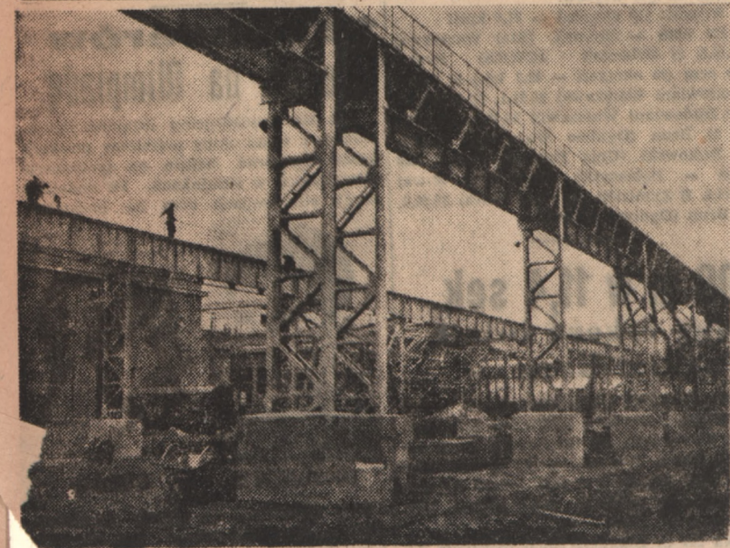
Nowej Hucie został już częściowo zmontowany nowoczesny transport międzyhalowy produkcji radzieckiej. Na zdjęciu: przodujący monterzy z brygady Tadeusza Bala sprawdzają montaż transportera. (CAF — fot. Baranowski)
