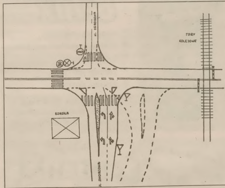
Rys. Skrzyżowanie Dworcowa - Mickiewicza. Propozycja zmiany geometrii skrzyżowania przy średnich nakładach finansowych (linią przerywaną oznaczono układ dotychczasowy).
