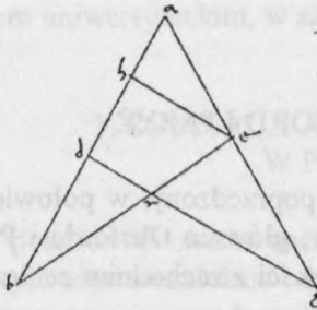
Ryc. 1. Narzędzia matematyczne astronomii: „linie (cięciwy) w kole” oraz sector figurae Menelaosa, dowód z połowy XV w.
