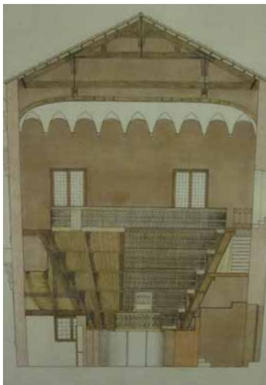
Przekrój architektoniczny przedstawiający schemat budowy „Teatru Anatomicznego”
